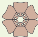
Габаритні розміри: 1600x1526 мм
